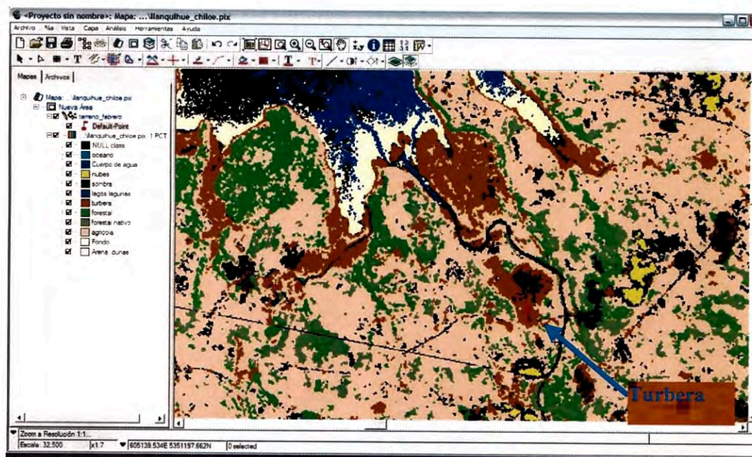
Imagen n° 2: Clasificación supervisada, Imagen Aster zona de Ancud.
